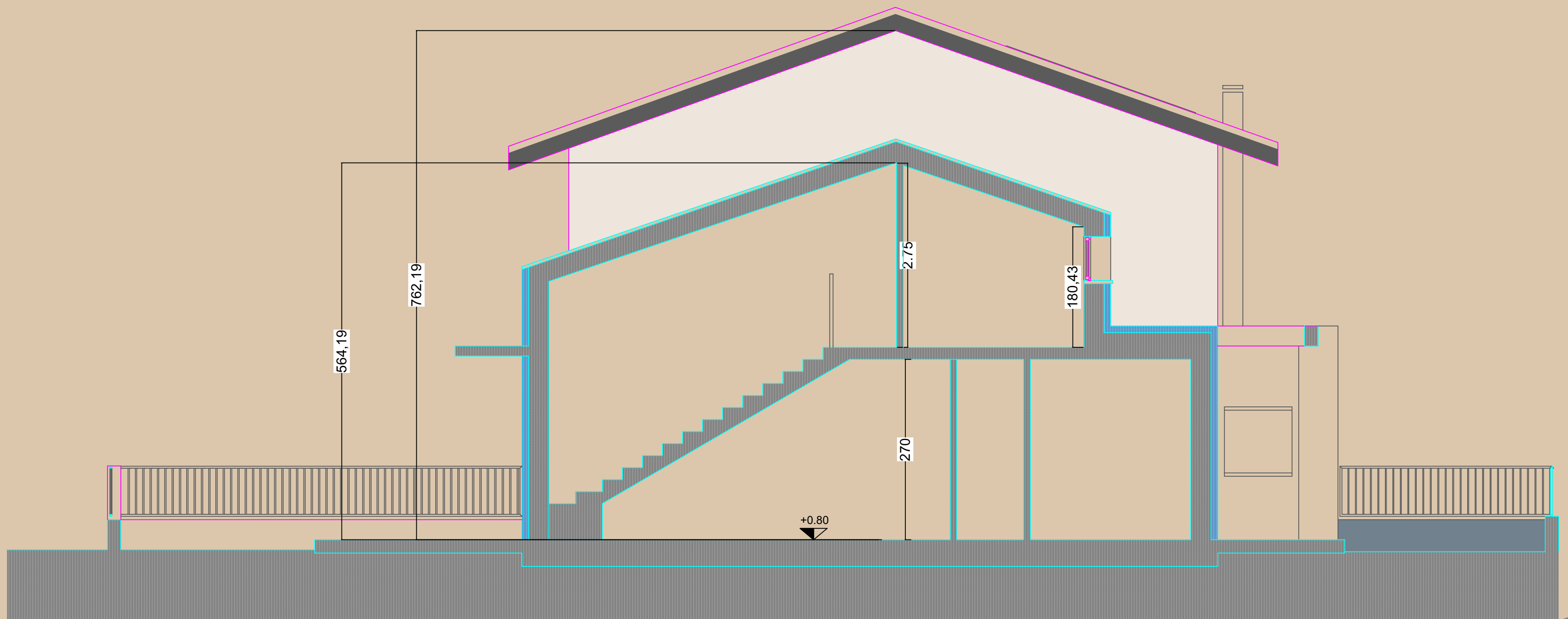
SEZIONE B-B
