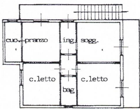
Pianta piano primo h.300
